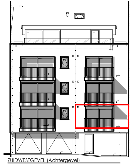
ZUIDWESTGEVEL (Achtergevel)
