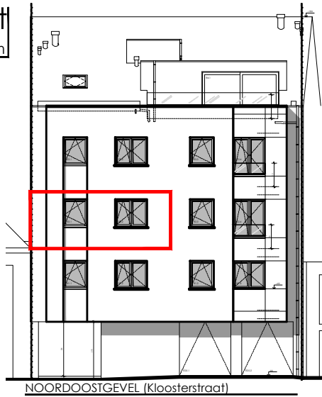
NOORDOOSTGEVEL (Kloosterstraat)
