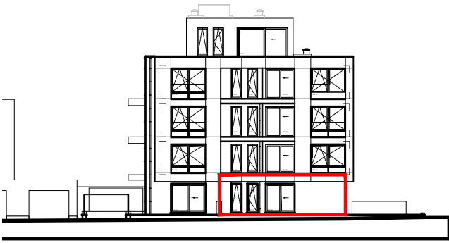
ZUIDGEVEL (Groeneweg)
